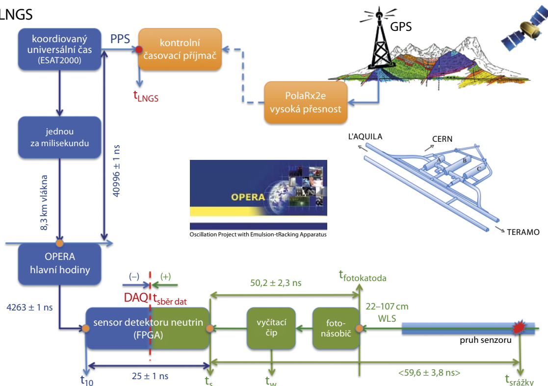
Obr. 1 Schéma časovacího systému experimentu OPERA v LNGS. Modře označená zpoždění oproti okamžiku srážky v detektoru mají tu vlastnost, že při jejich růstu se \delta t zmenšuje, zatímco při růstu zeleně označených zpoždění \delta t roste. Převzato z [2].
